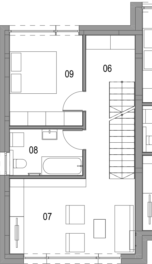
TLORIS NADSTROPJA
