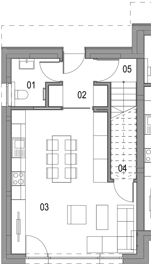
TLORIS PRITLIČJA
