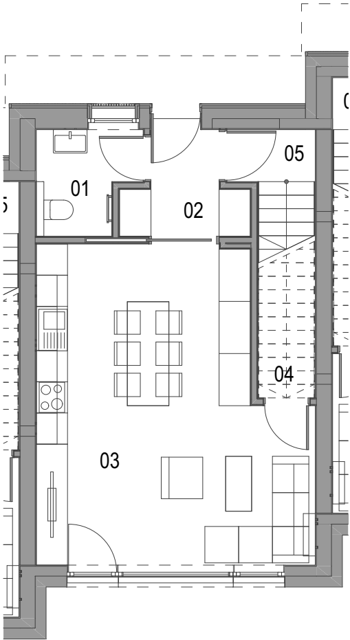
TLORIS PRITLIČJA
